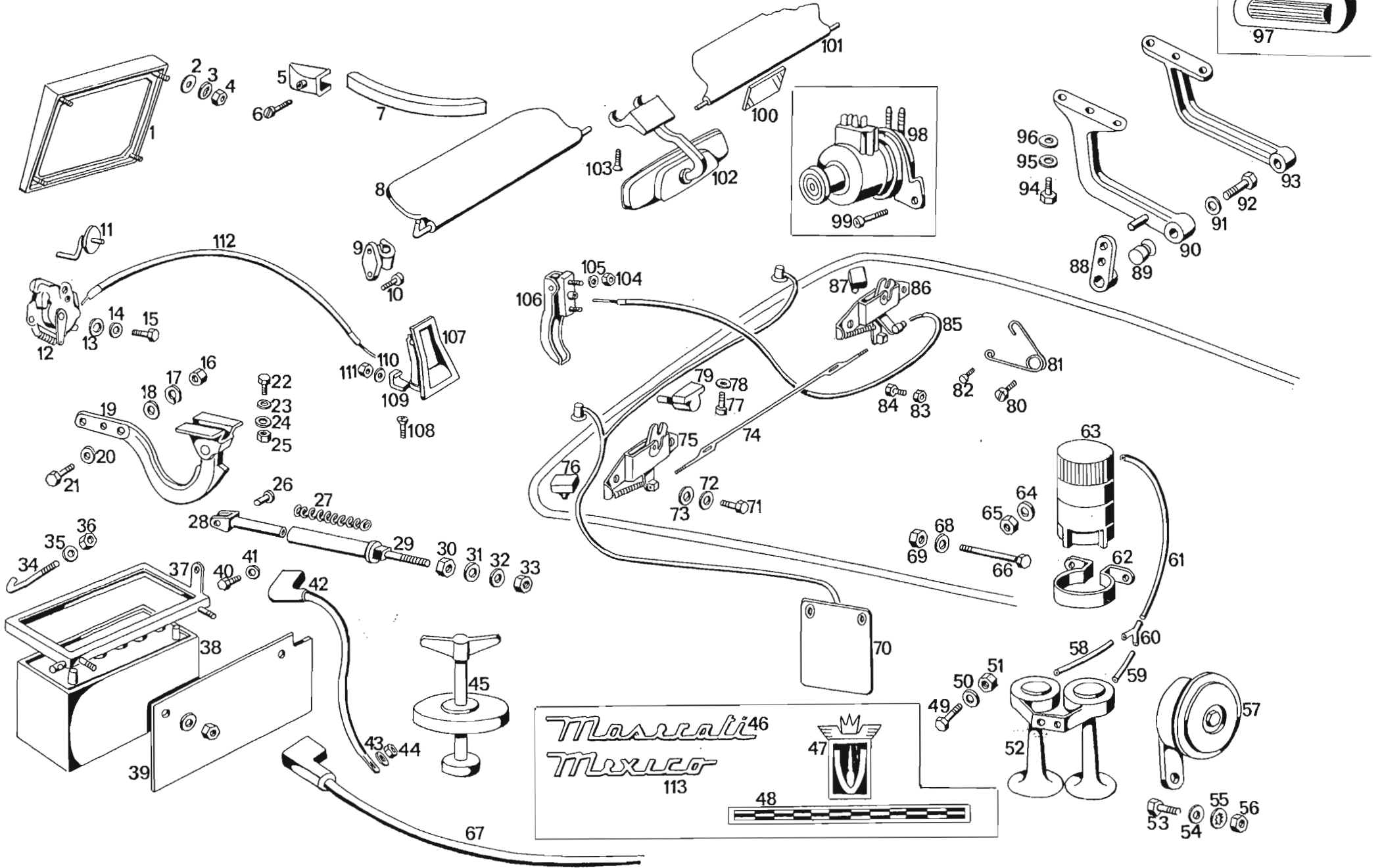
TAVOLA 7-VANO MOTORE E BAULE TABLEAU 7-COFFRE MOTEUR ET COFFRE À BAGAGES TABLE 7-ENGINE AND TRUNK COMPARTMENT TAFEL 7-MOTOR HAUBE UND KOFFERRAUM
